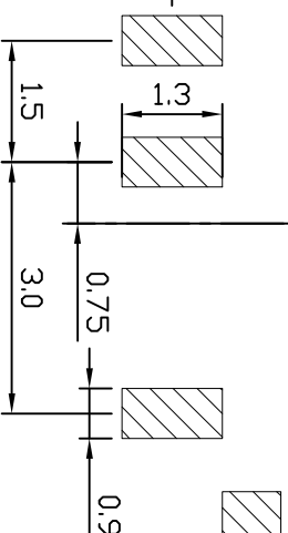
P.C.B LAYOUT
